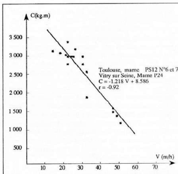
Figure 4 : Corrélation C-V obtenue dans les marnes en jumelant 3 forages sur les sites de Toulouse et de Vitry.
