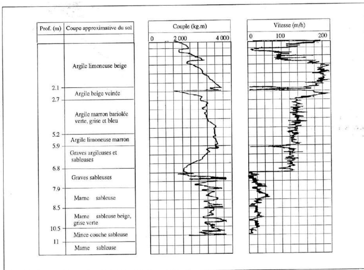
Figure 1 : Enregistrement des deux paramètres de forage couple et vitesse d'avancement avec le dispositif STARSOL-ENBESOL.
