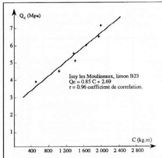
Figure 3 : Corrélation spécifique "Qc-C" obtenue dans une couche de limon du site Issy les Moulineaux.
