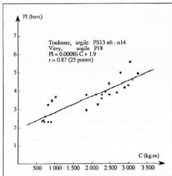
Figure 2 : Corrélation Pl-C obtenue dans les argiles en jumelant 3 forages sur les sites de Toulouse et de Vitry.
